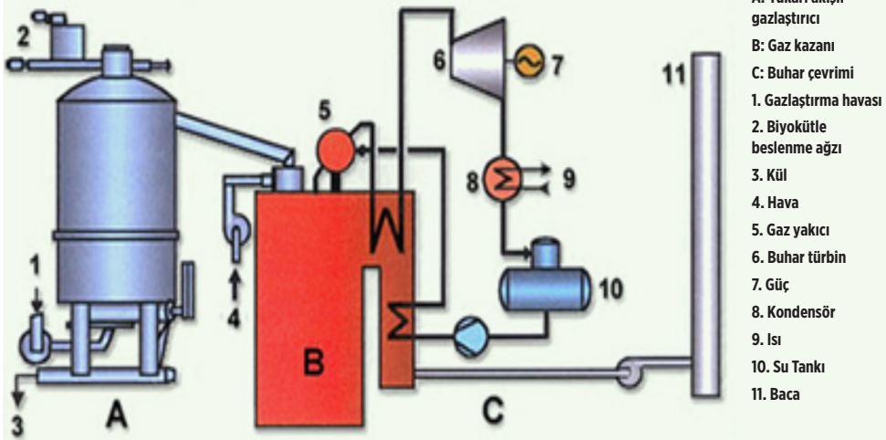
Şekil 64: Sabit Yataklı Gazlaştırıcı [1,5]
