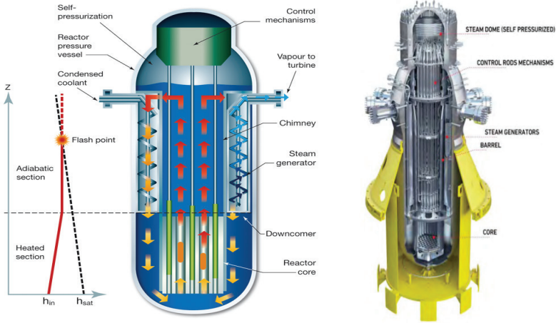
Şekil 4.5: CAREM Tasarımı [4.14, 4.15]
