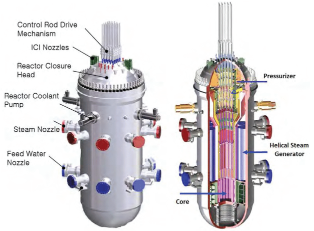
Şekil 4.31: SMART reaktör tasarımı [4.32]
