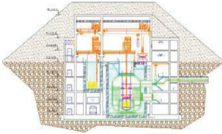
Şekil 4.27: Nuward tipik nükleer ada kesiti [4.25].
