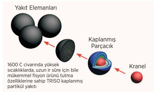
Şekil 4.18: TRISO yakıt [4.8]
