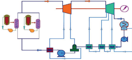
Şekil 4.17: HTR-PM santralının basit akış şeması [4.21]
