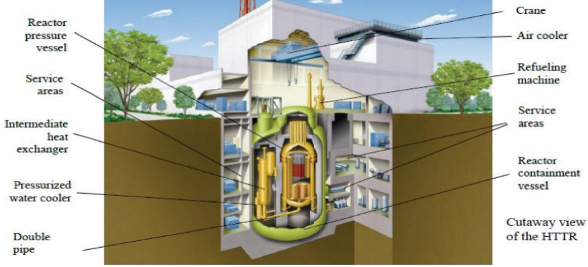
Şekil 4.43: HTTR30 tasarımı genel görünüm [4.44]
