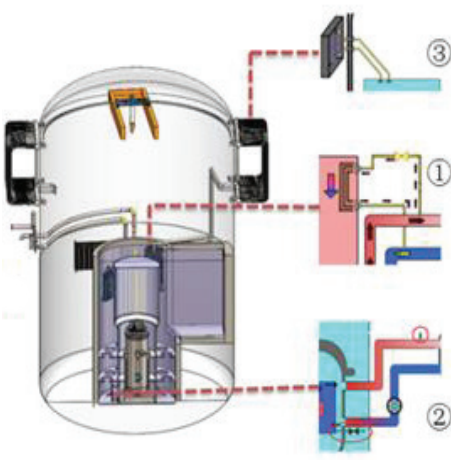
Şekil 4.10: HAPPY-200 tasarlanmış güvenlik özellikleri: (1) pasif buharlaşma ısı giderme sistemi, (2) pasif güvenlik enjeksiyon sistemi, (3) pasif hava soğutma sistemi [4.8]
