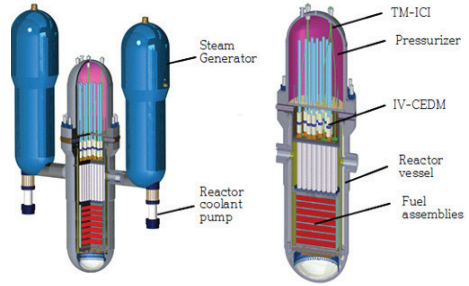
Şekil 4.33: BANDI-60S tasarımının temsili görünümü [4.34]
