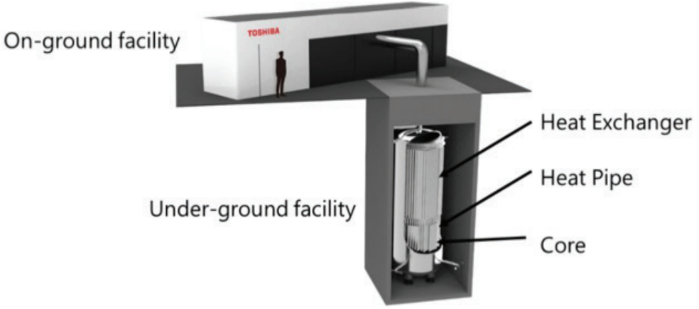
Şekil 4.46: MoveLux tasarımının genel görünümü [4.48]
