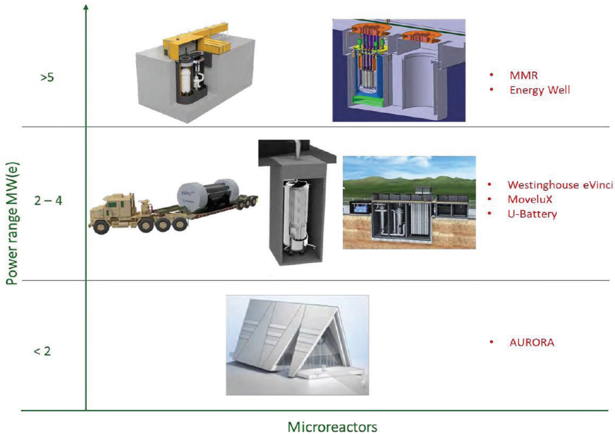
Şekil 3.9: Bazı mikro-reaktörler [3.18]
