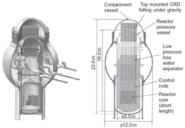
Şekil 4.39 CCR tasarımı genel görünüm [4.44]
