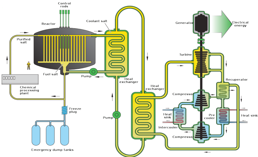
Şekil 3.8: Ergimiş tuz reaktörü (MSR) şeması [3.15].
