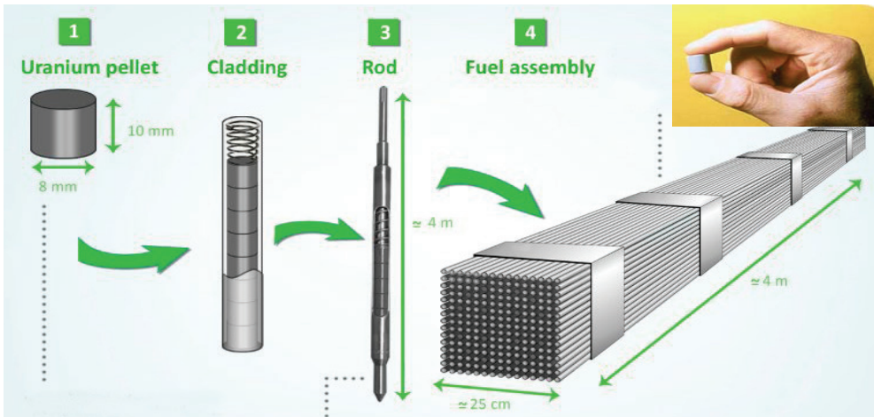
Şekil 1.2: İşlenmiş Uranyum (Yakıt çubukları) [1.4, 1.5]
