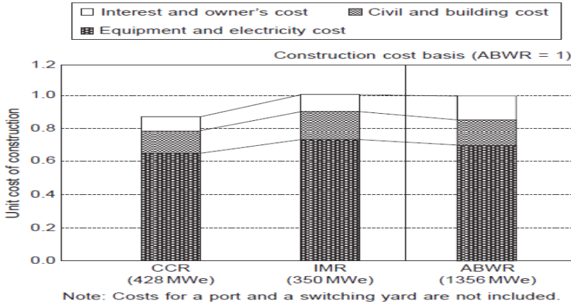
Şekil 4.40: IMR ve CCR'nin inşaat maliyeti değerdendirmesi [4.44]
