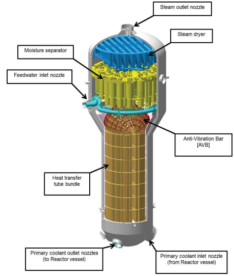
Şekil 1.4: Buhar üretici [1.8, 1.11]
